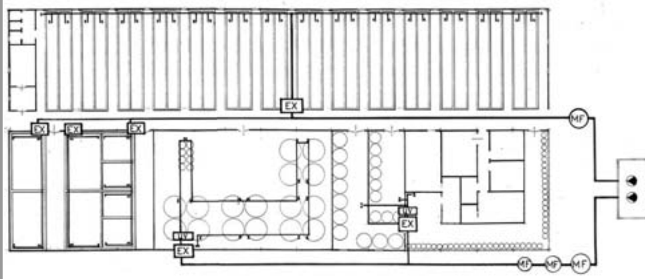
Fig. 49 - Hatchery circuits
