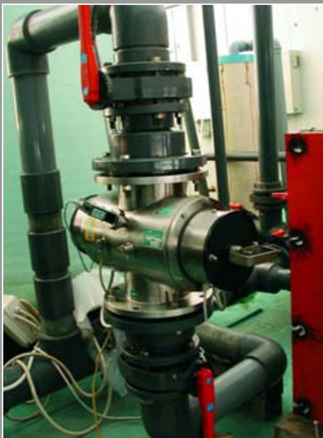
Fig. 70 - UV lamp
